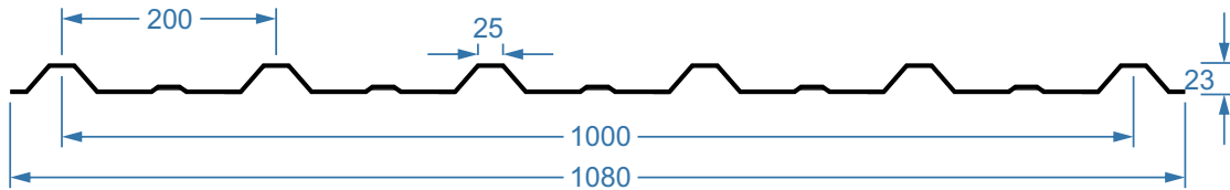
Hình ảnh cấu tạo sóng theo mặt cắt Tấm lợp Eurolines 6 sóng / Image composition waves in sectional
